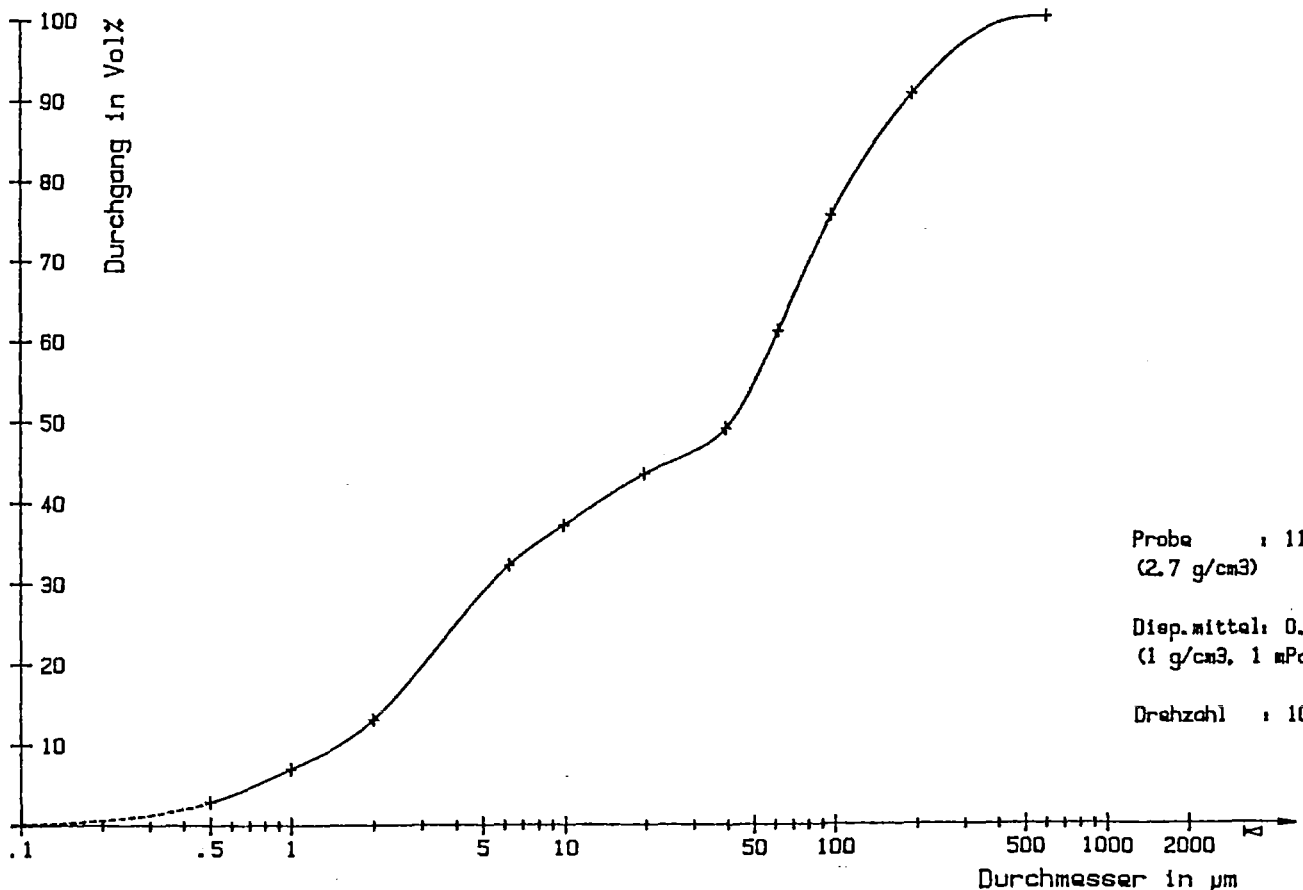
Teilchengroessenverteilung
