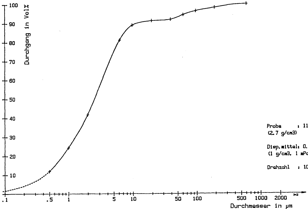
Teilchengrößenverteilung
