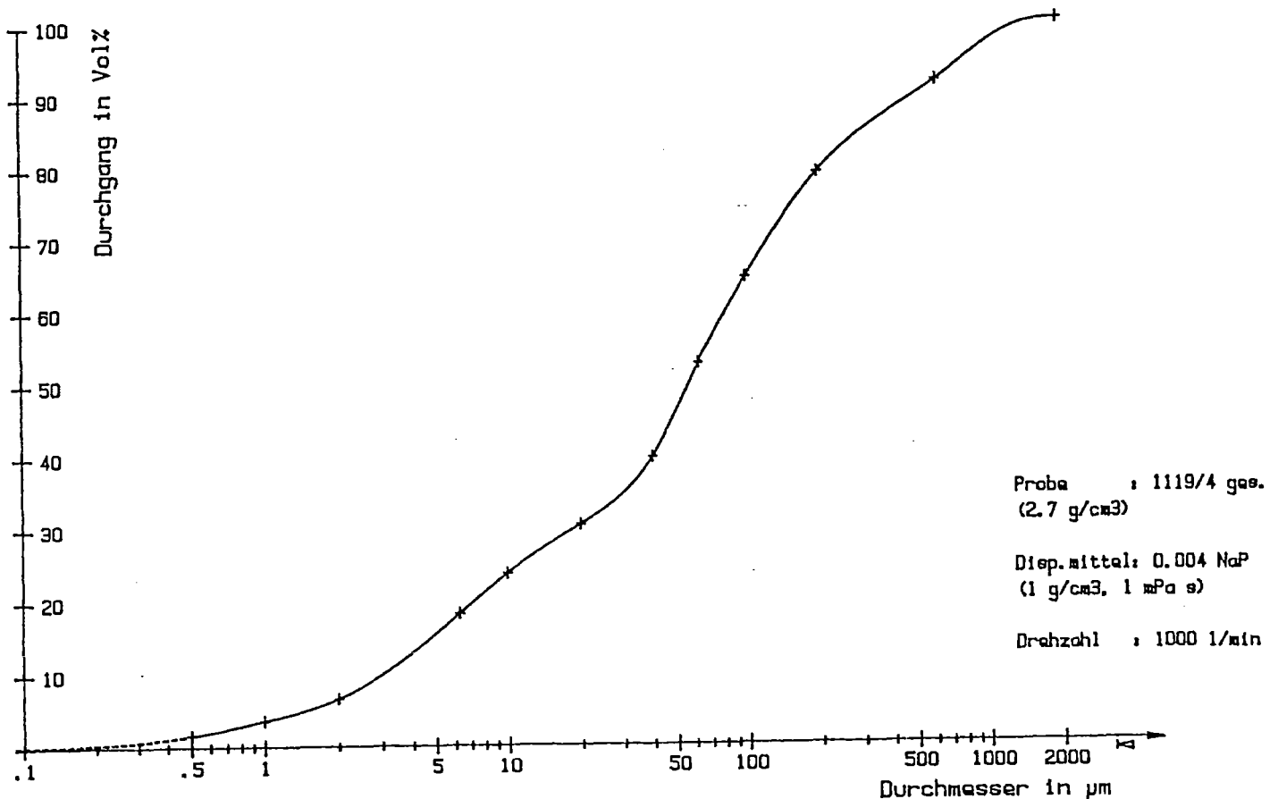
Teilchengrossenverteilung
